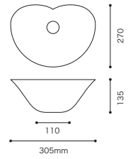
だ円変形 DH - D27
