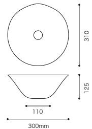
丸鉢排水栓 PH31-25
