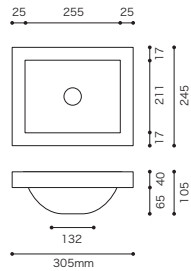
長角 W30×D24 埋め込み
