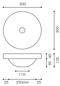
30φ丸埋め込み
